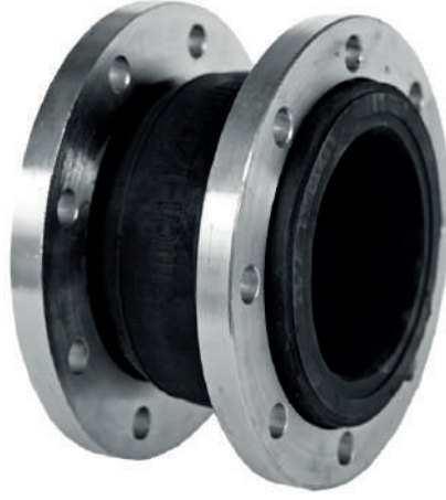
Flanşlı Kauçuk Kompansatör Flanged Rubber Expansion Joint
